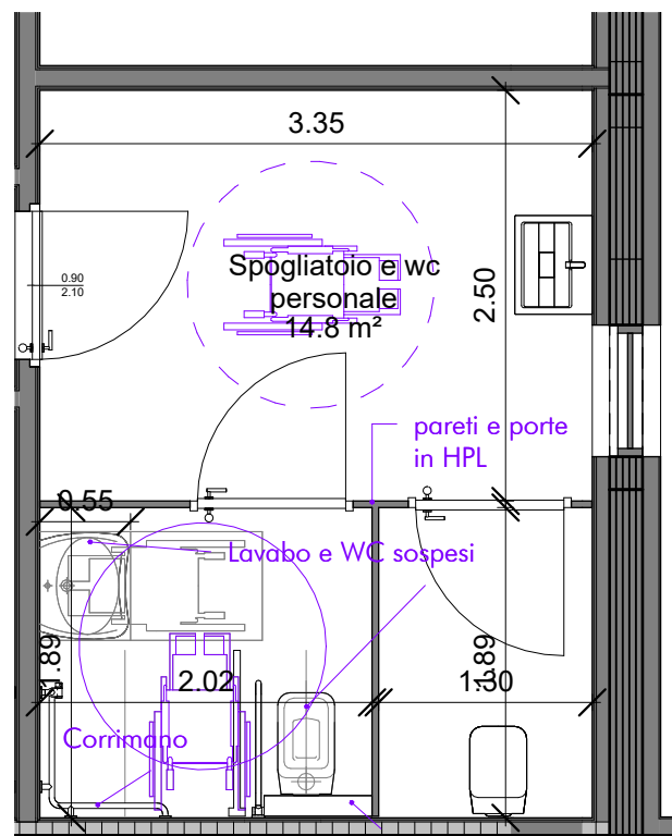
SPOGLIATOIO E WC PERSONALE
