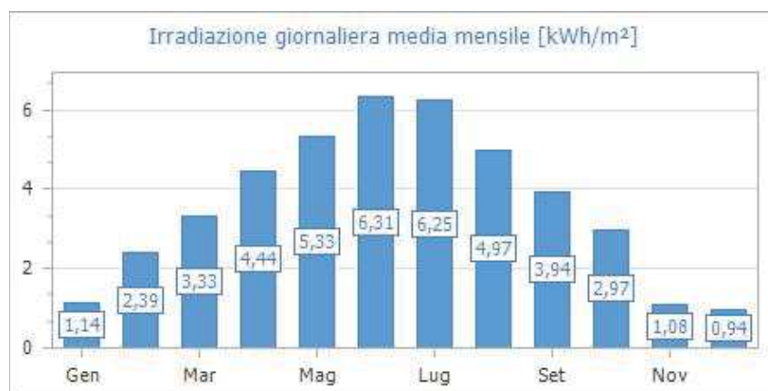
Fig. 1: Irradiazione giornaliera media mensile sul piano orizzontale [kWh/m 2 ]- Fonte dati: UNI 10349:2016 - Stazione di rilevazione: Vertemate con Minoprio
