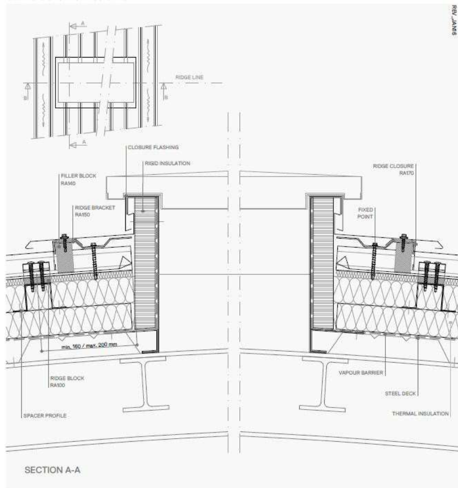
DETTAGLIO TIPO RIVERCLACK NODO COERTURA-GRONDA
